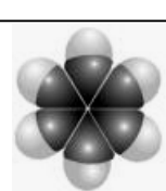
苯分子图
